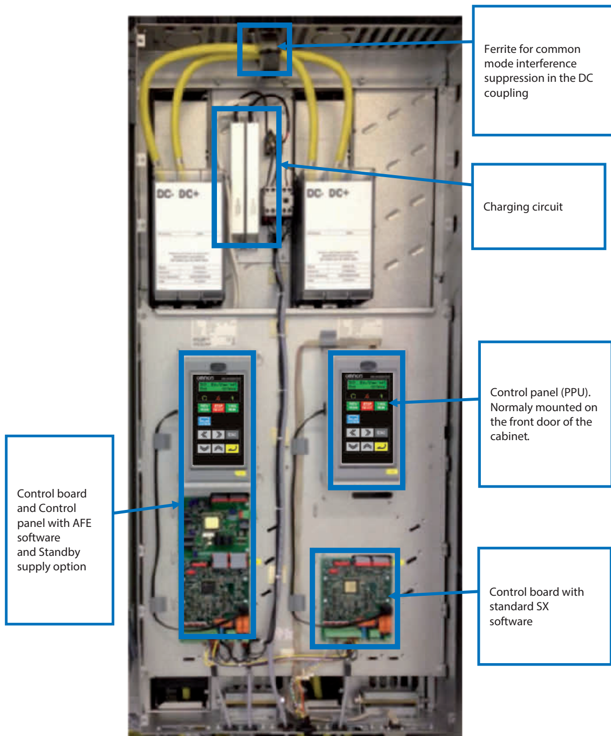
Fig. 24 AFE + VSI
