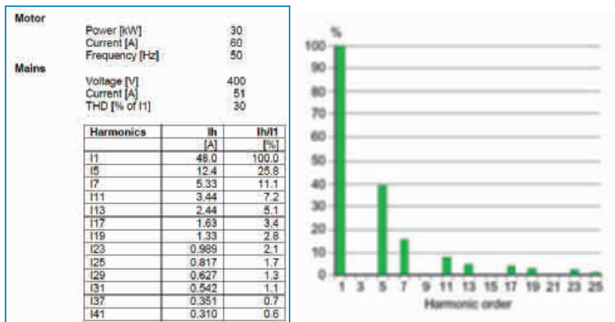
Fig. 4 THDI
