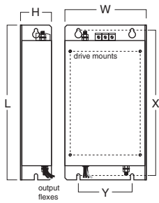
Footprint dimensions
