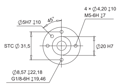
Gripper dimensions
