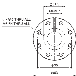
Gripper dimensions
